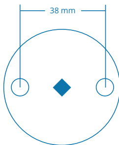
Euroopa standardi kinnitus (E) 38mm
